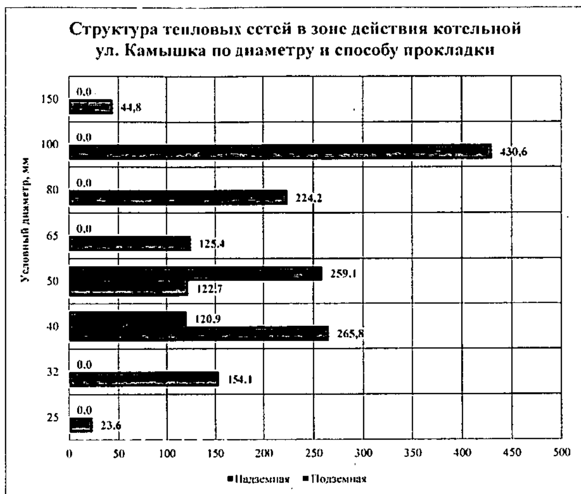
Рисунок 9 – Структура тепловых сетей в зоне действия котельной «Камышка»
