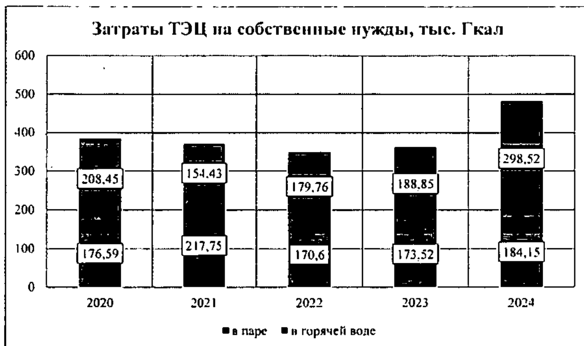
Рисунок 16 – Динамика изменения затрат тепловой энергии на собственные нужды ТЭЦ АО «РИР»
