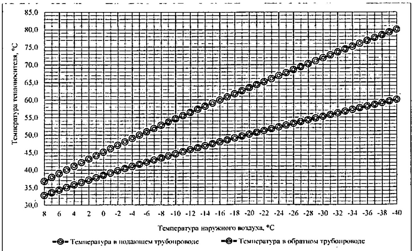
Рисунок 13 – Температурный график режима работы котельной «Камышка»
