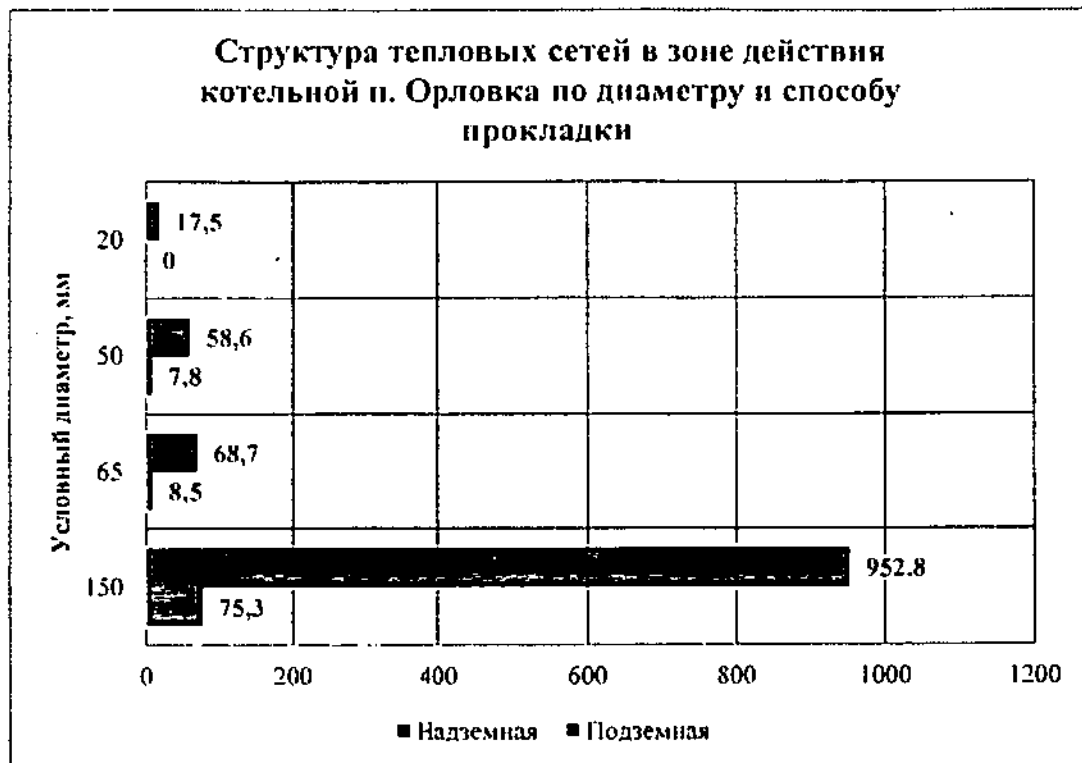
Рисунок 10 – Структура тепловых сетей в зоне действия котельной п. Орловка
