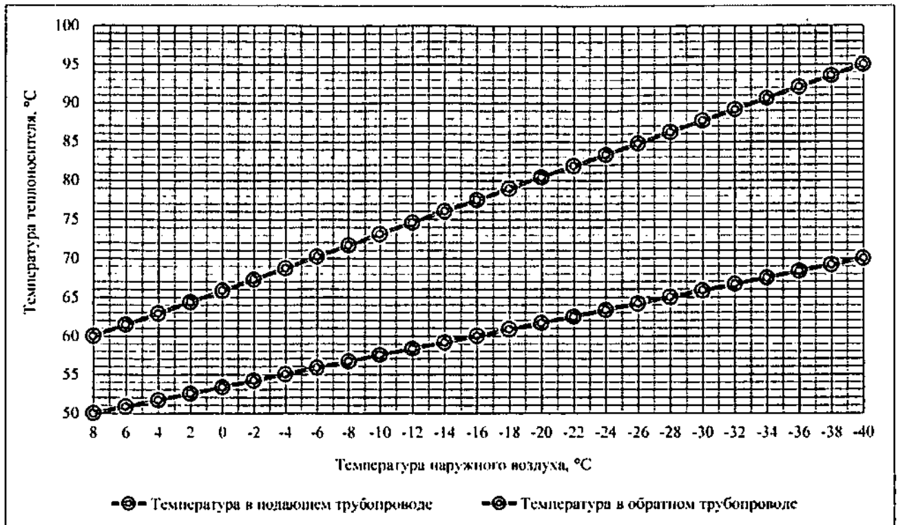
Рисунок 12 – Температурный график режима работы котельной «ЦОК»
