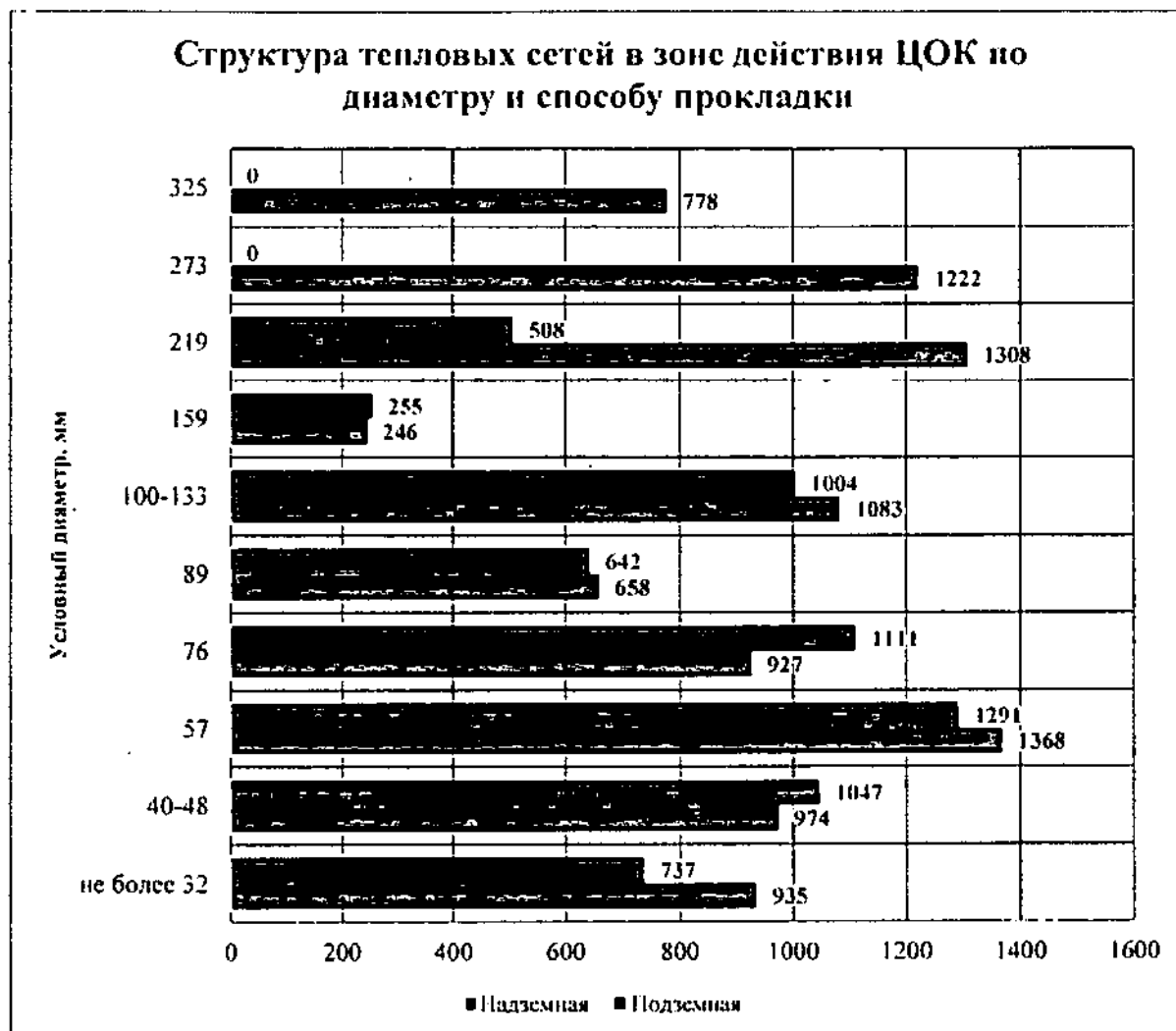
Рисунок 8 – Структура тепловых сетей в зоне действия котельной «ЦОК»
